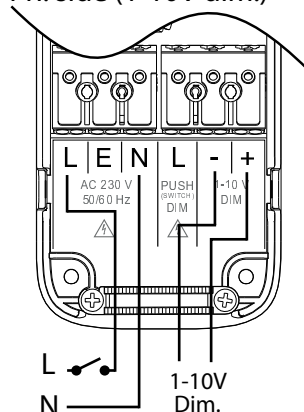
Pri. side (1-10V dim.)
