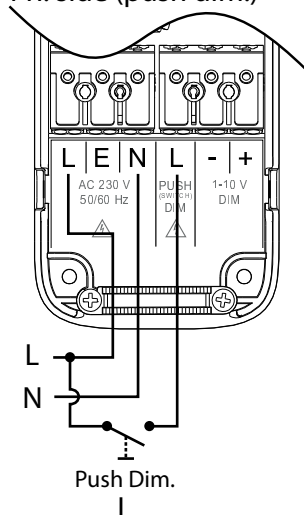
Pri. side (push dim.)
