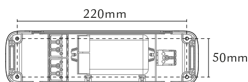
Pri. side (push dim.)
